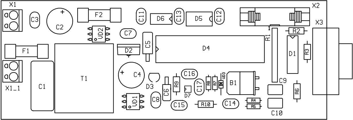
Элементы стороны Тор платы DEMO. Плата показана со стороны Тор.
