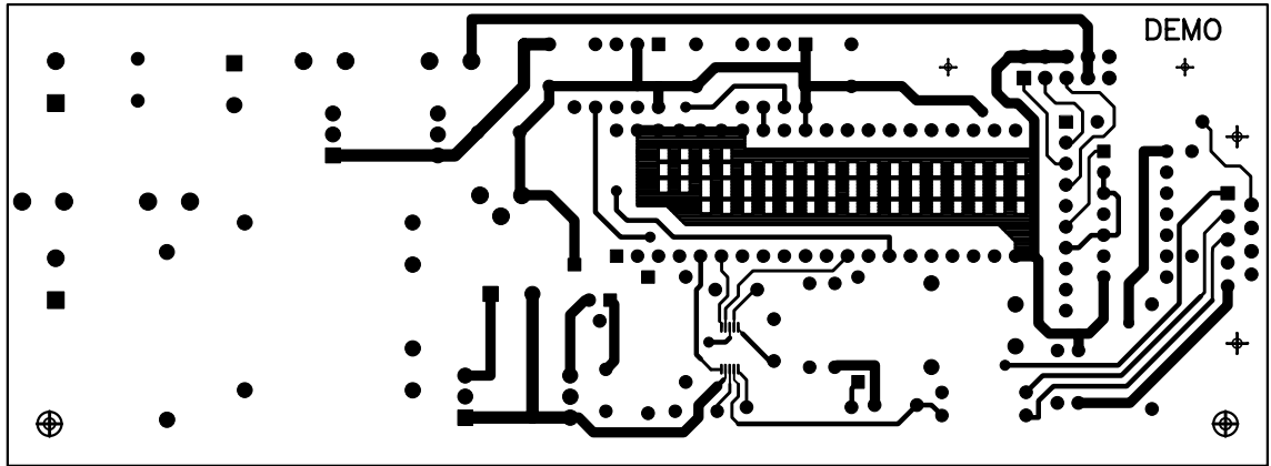
Сторона Top платы DEMO. Плата показана со стороны Top.
